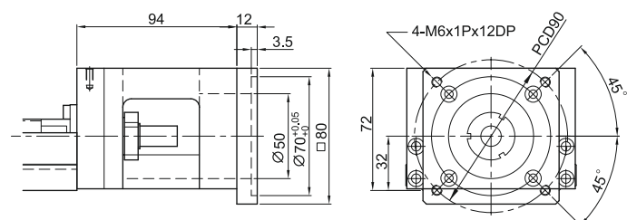
Moduł KK100 Kołnierz łączący F1
