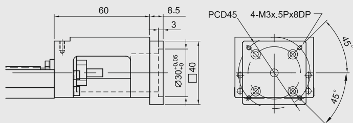
Moduł KK50 Kotłnierz łączący F2
