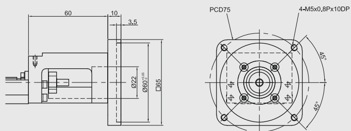
Moduł KK50 Kotłnierz łączący F6
