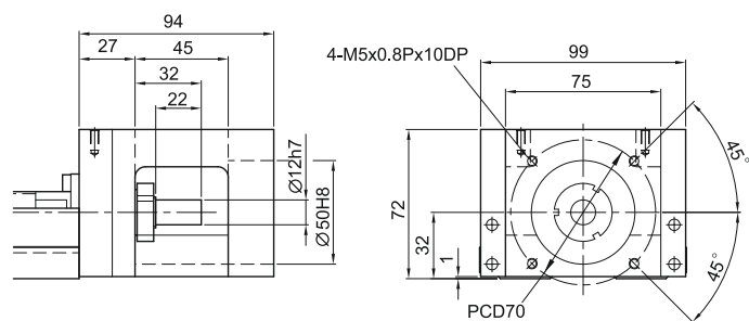
Moduł KK100 Kołnierz łączący F0
