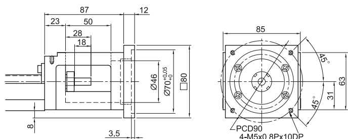
Moduł KK86 Kołnierz łączący F4
