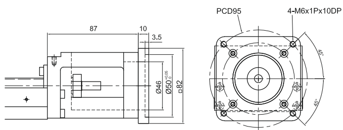
Moduł KK86 Kołnierz łączący F10
