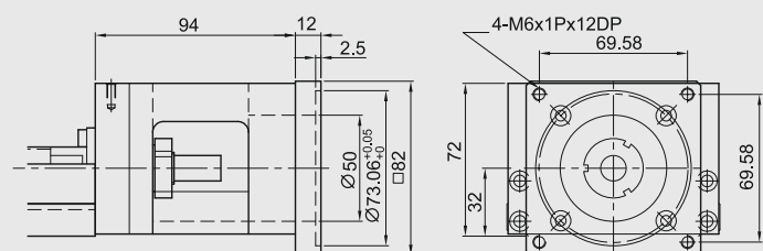
Moduł KK100 Kołnierz łączący F4
