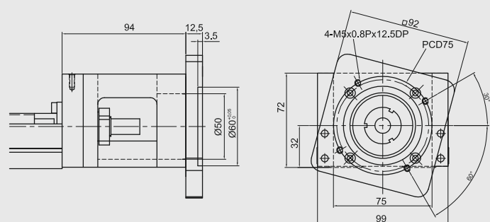
Moduł KK100 Kołnierz łączący F6
