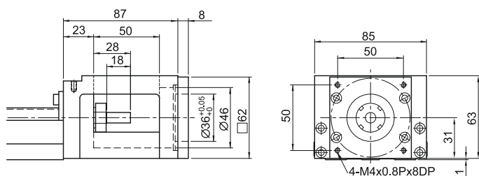
Moduł KK86 Kołnierz łączący F5
