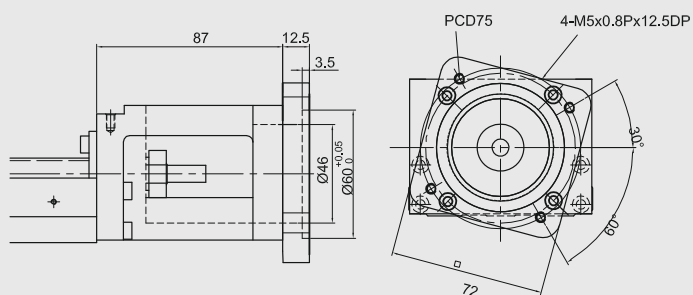
Moduł KK86 Kołnierz łączący F8
