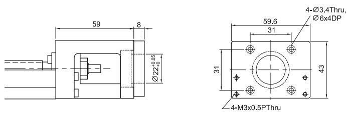
Moduł KK60 Kołnierzy łączący F5
