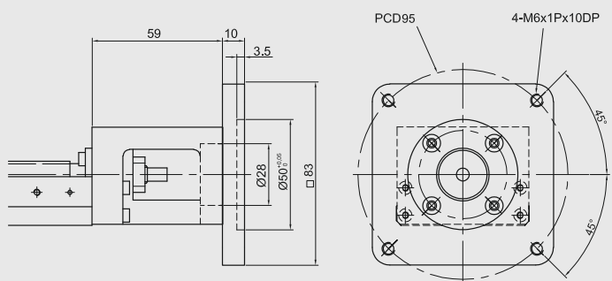
Moduł KK60 Kołnierzy łączący F9
