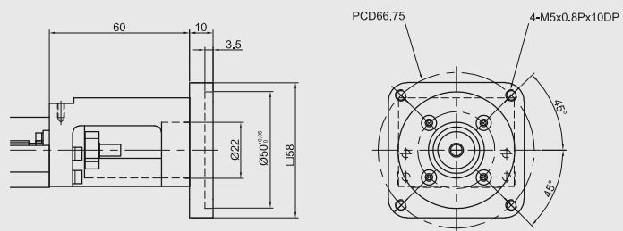
Moduł KK50 Kotłnierz łączący F7
