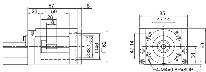
Moduł KK86 Kołnierz łączący F6
