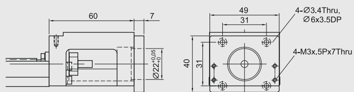
Moduł KK50 Kotłnierz łączący F3
