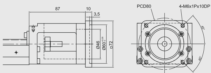
Moduł KK86 Kołnierz łączący F9
