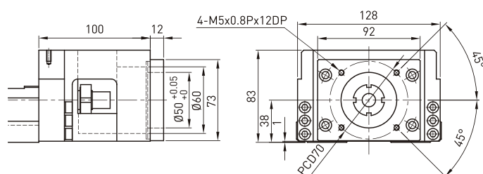
Moduł KK130 Kołnierz łączący F1
