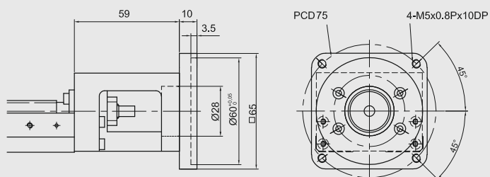
Moduł KK60 Kołnierzy łączący F10
