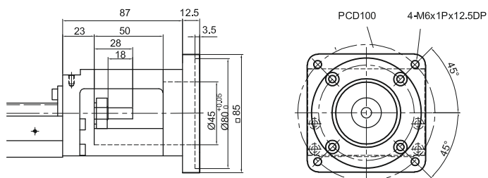
Moduł KK86 Kołnierz łączący F7
