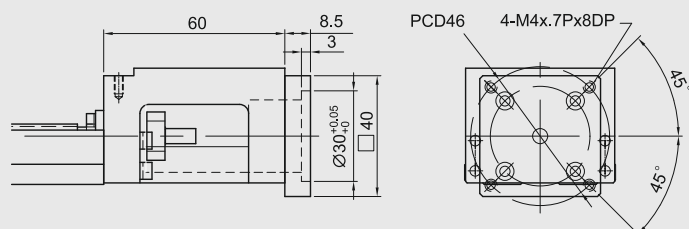
Moduł KK50 Kotłnierz łączący F1
