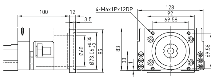
Moduł KK130 Kołnierz łączący F3
