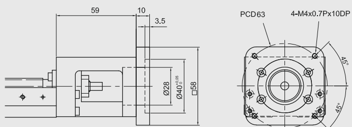
Moduł KK60 Kołnierzy łączący F8
