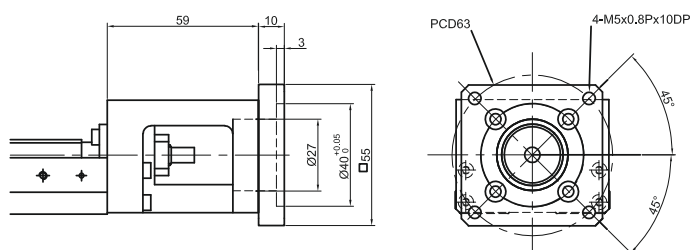
Moduł KK60 Kołnierzy łączący F6
