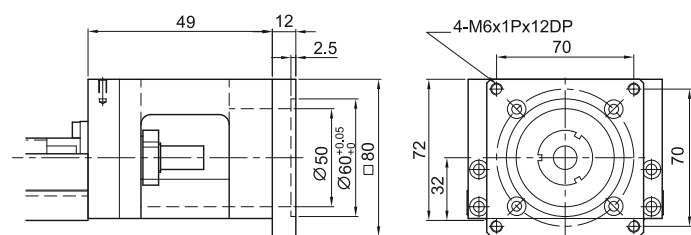
Moduł KK100 Kołnierz łączący F3
