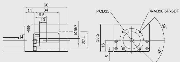
Moduł KK50 Kotłnierz łączący F0
