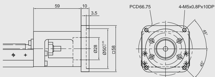
Moduł KK60 Kołnierzy łączący F11
