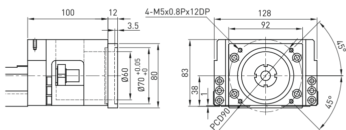
Moduł KK130 Kołnierz łączący F4
