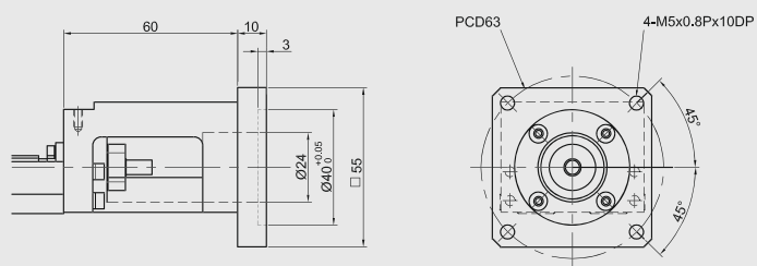
Moduł KK50 Kotłnierz łączący F4
