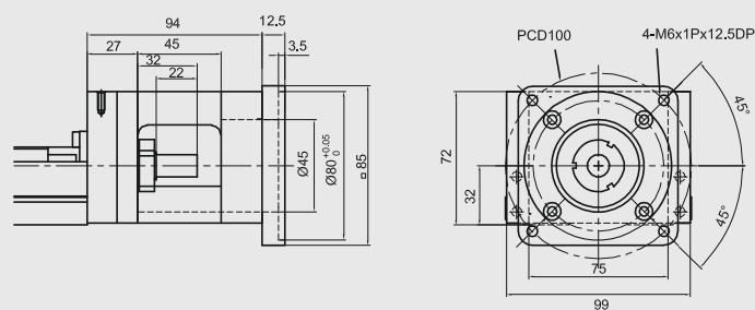
Moduł KK100 Kołnierz łączący F5
