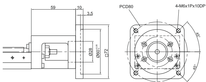
Moduł KK60 Kołnierzy łączący F7
