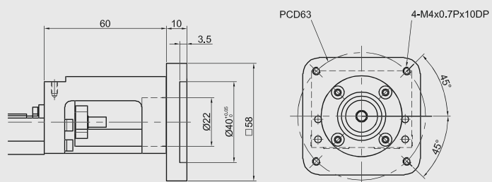
Moduł KK50 Kotłnierz łączący F5
