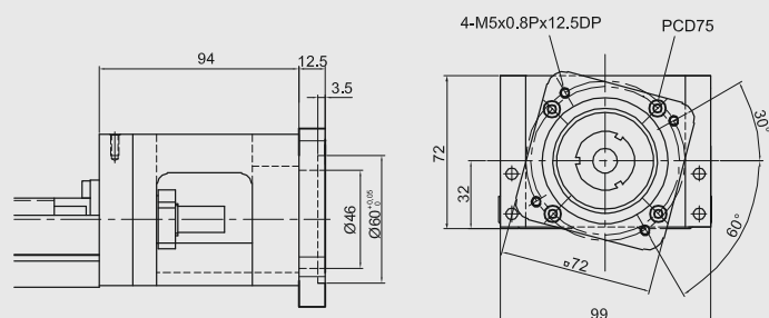
Moduł KK100 Kołnierz łączący F7
