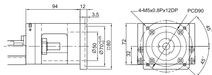
Moduł KK100 Kołnierz łączący F2
